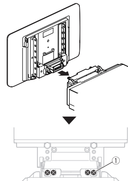
① Stelschroef (4 mm × 6 mm)
